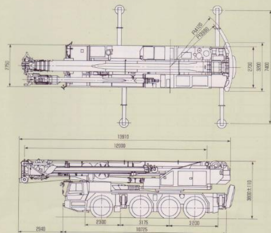
■外観寸法図
